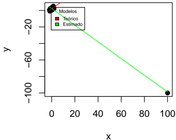
Figura 12.4: Modelo con 1 outlier
