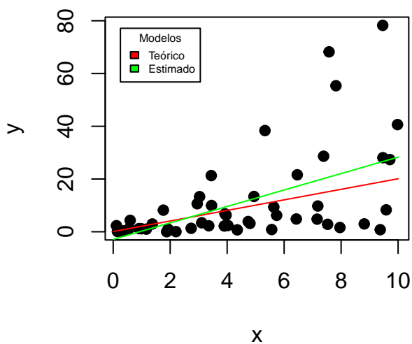
Figura 12.5: No se cumple la hipótesis de que los errores sean normales
