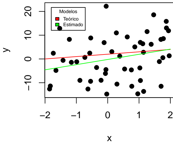
Figura 12.2: El valor \sigma del desvío de los errores es grande.
