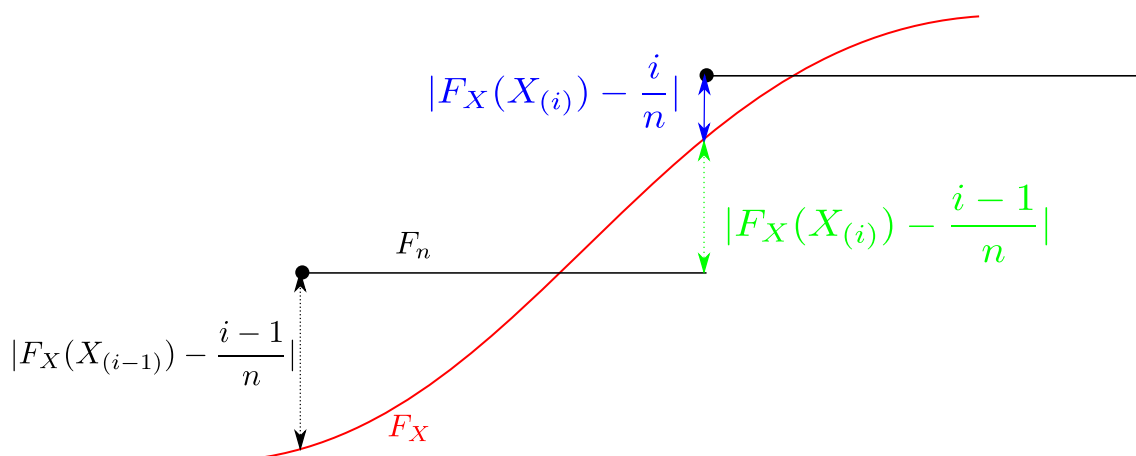
Figura 10.1: En rojo se grafica la función de distribución F_X en negro la distribución empírica F_n . En azul se muestra |F_X(X_{(i)}) - \frac{i}{n}| y en verde |F_X(X_{(i)}) - \frac{i-1}{n}|
