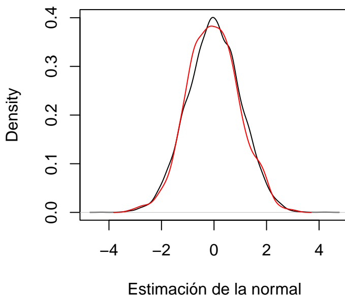
Figura 4.4: Estimación de la densidad normal con media 0 y varianza 1 con 10000 datos (en negro) y con 1000 datos (en rojo)
