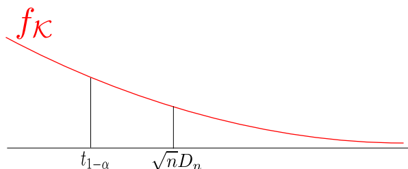
Figura 10.3: En rojo se grafica la densidad de la variable \mathcal{K} , si el área desde t_{1-\alpha} en adelante es \alpha , y el área desde \sqrt{n}D_n (el cual es por definición el p -valor) es menor que \alpha esto implica que \sqrt{n}D_n > t_{1-\alpha} y por lo tanto se rechaza H_0 .
