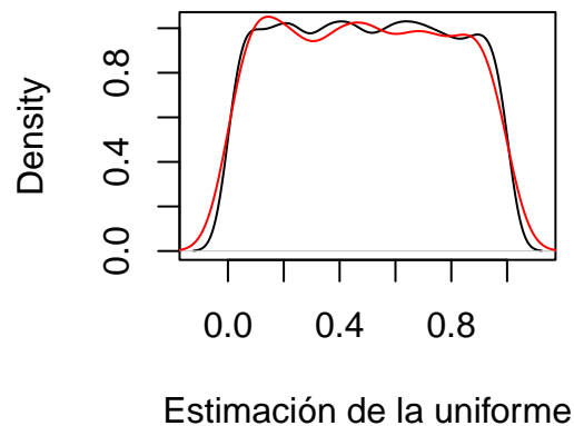
Figura 4.3: Estimación de la densidad uniforme con 10000 datos (en negro) y con 1000 datos (en rojo)
