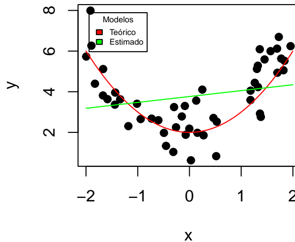
Figura 12.3: Hay una relación no lineal entre las variables
