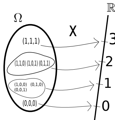
Figura 3.1: Variable aleatoria Binomial en el caso de 3 experimentos
