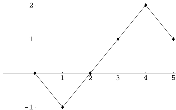
Figura 1: Una trayectoria del paseo al azar
