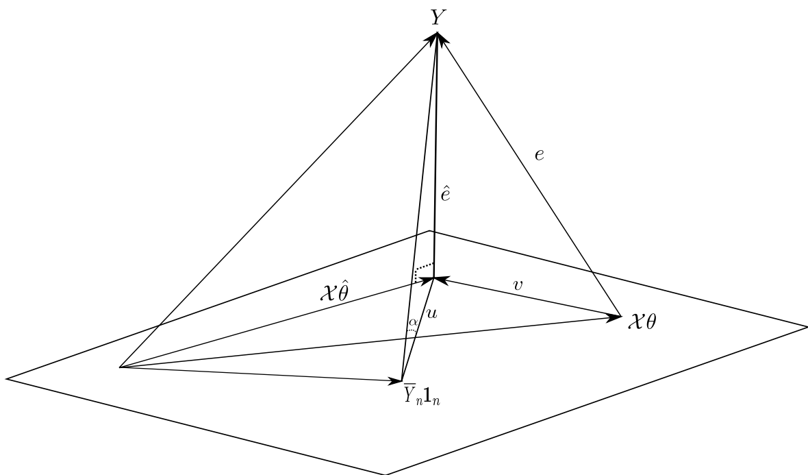
Figura 7.1: X_{\hat{\theta}} es la proyección ortogonal de Y sobre el espacio generado por las columnas de X . \mathbf{1}_n = (1, 1, \dots, 1) \in \mathbb{R}^n . R^2 = \cos(\alpha) . Observar que \|u\|^2 = SC_{Reg}
