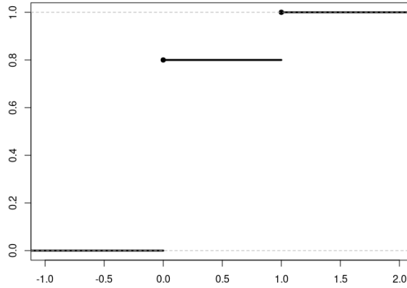
Figura 2.4: Gráfico de la función de distribución de una variable X \sim \text{Ber}(0,2) .
