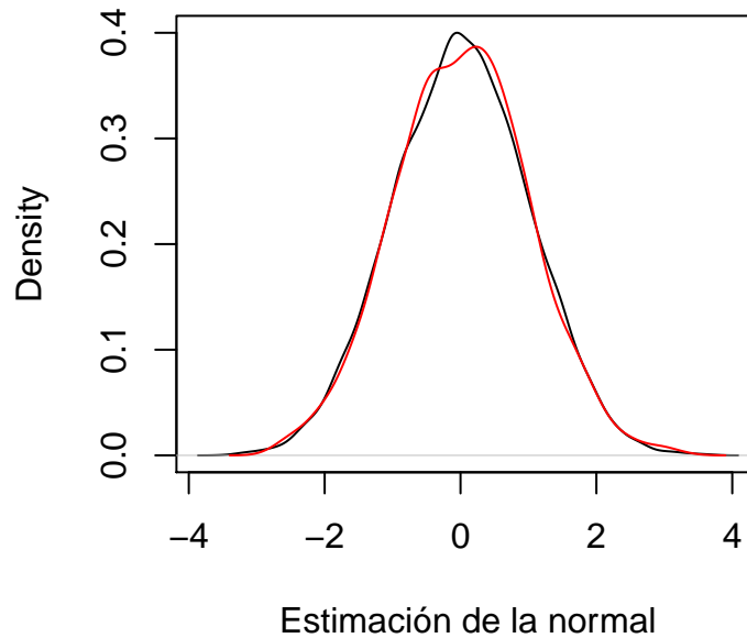
Figura 2.6: Estimación de la densidad normal con media 0 y varianza 1 con 10000 datos (en negro) y con 1000 datos (en rojo)
