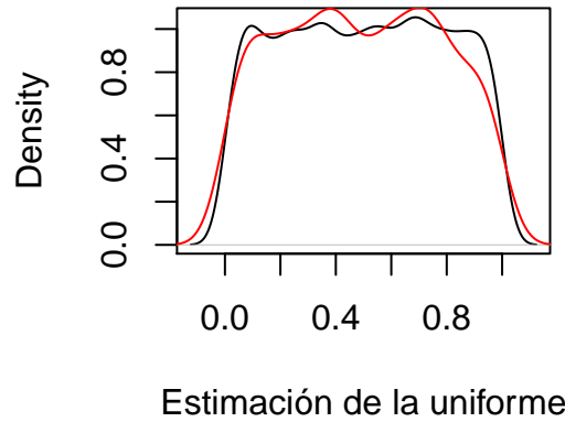
Figura 2.5: Estimación de la densidad uniforme con 10000 datos (en negro) y con 1000 datos (en rojo)
