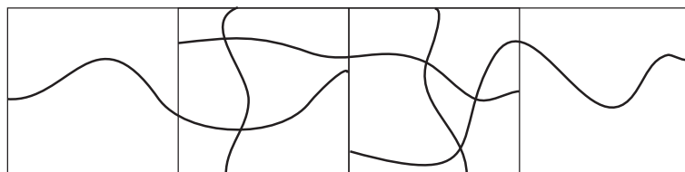
Figura 2.15: Tres 2n por n rectángulos y dos n cuadrados, dibujados con caminos que garantizan a un cruce horizontal de su unión.
