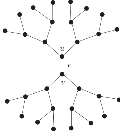
Figura 3.1: Una región del grafo \mathbb{T}_2 .
