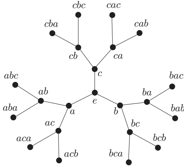
Figura 3.3: \mathbb{T}_2 es un grafo de Cayley
